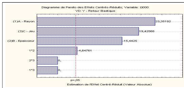
FIG. 5.5 – Diagramme de Pareto pour le retour élastique
