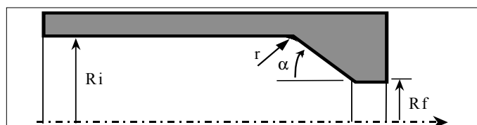
FIG. 5.10 – Modèle axisymétrique pour le processus d'extrusion.
