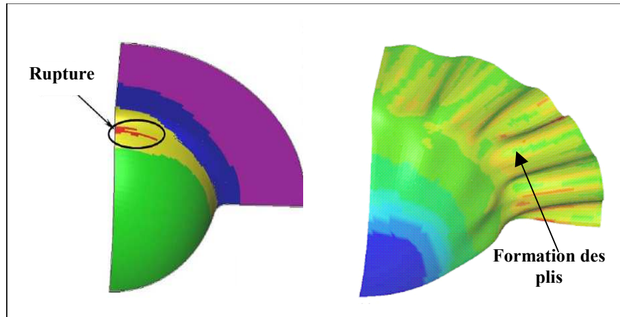
FIG. 1.16 – Simulation numérique des plis et de la rupture en hydroformage.
